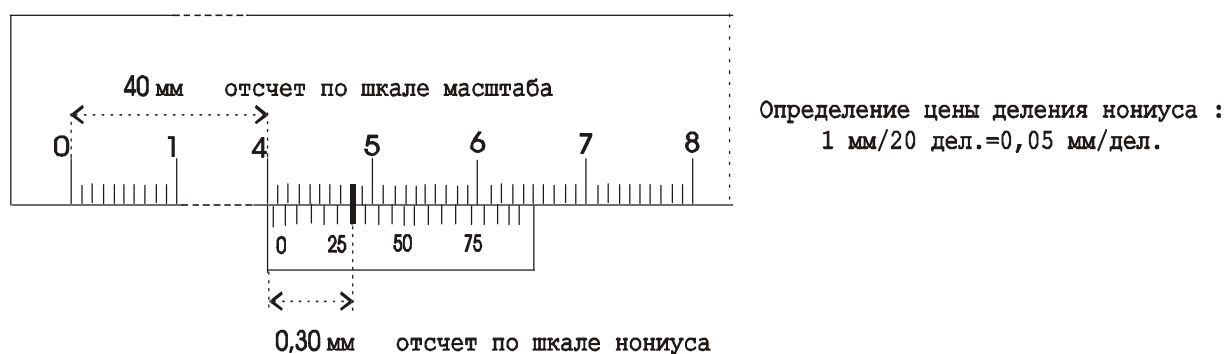
Рис.1.1. Штангенциркуль
