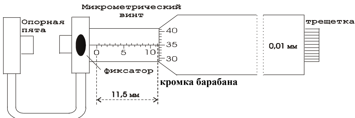
Рис.1.2 Микрометр
