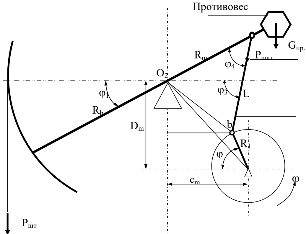
Рис. 2. Схема к расчету усилий
