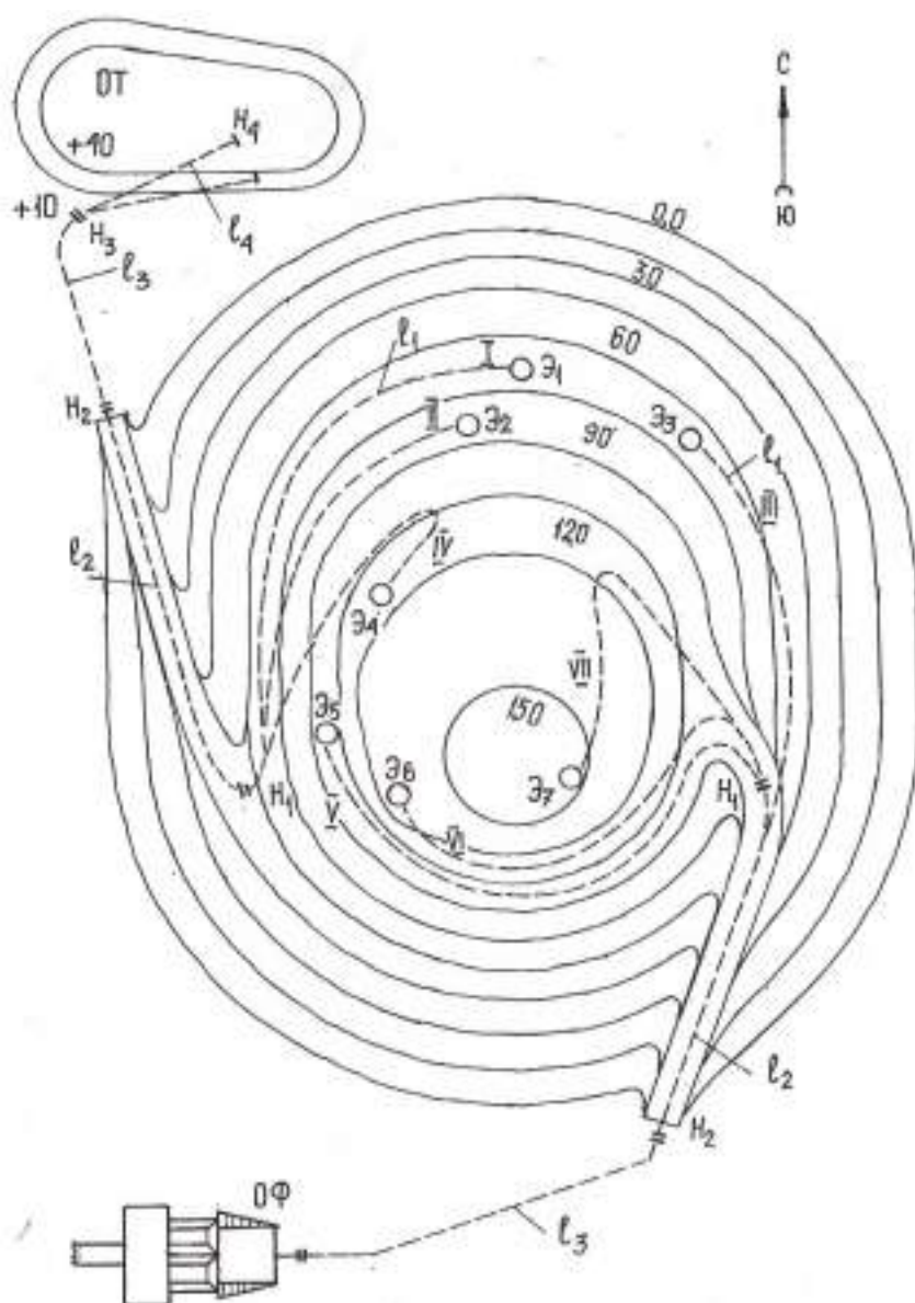
Рис. 3.2. План условного карьера
