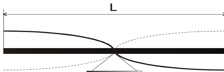
Рис. 5.1.Схема излучателя колебаний
