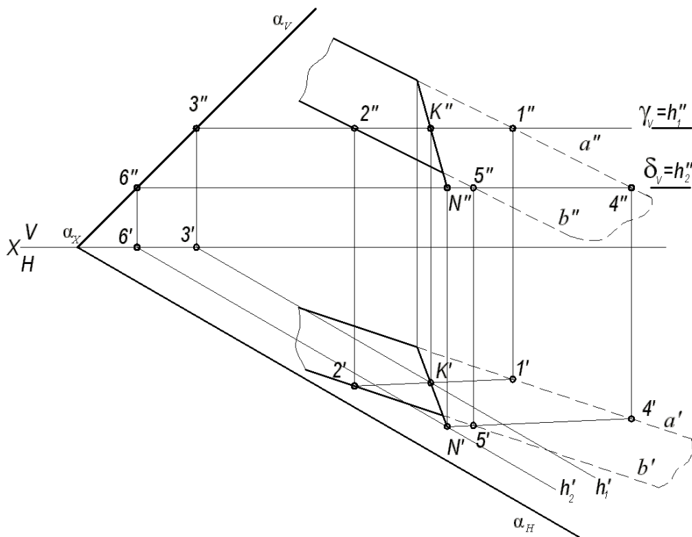
Рис. 5. Построение линии пересечения двух плоскостей
