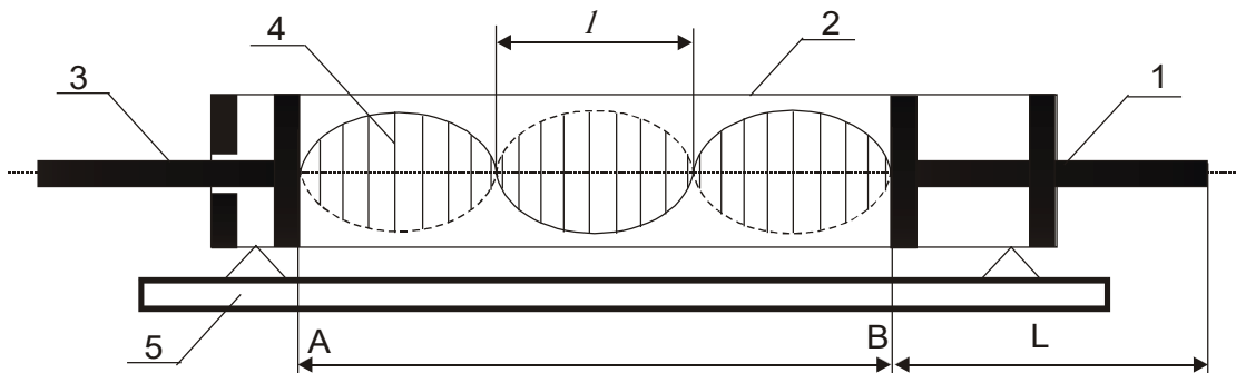
Рис.5.2. Схема установки :
