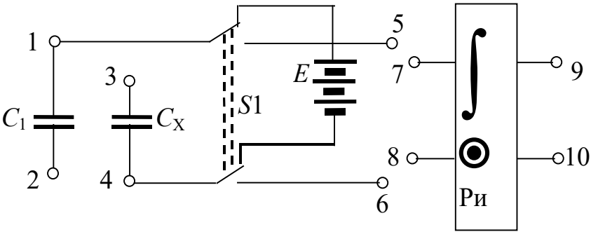
Рис.2. Схема экспериментальной установки
