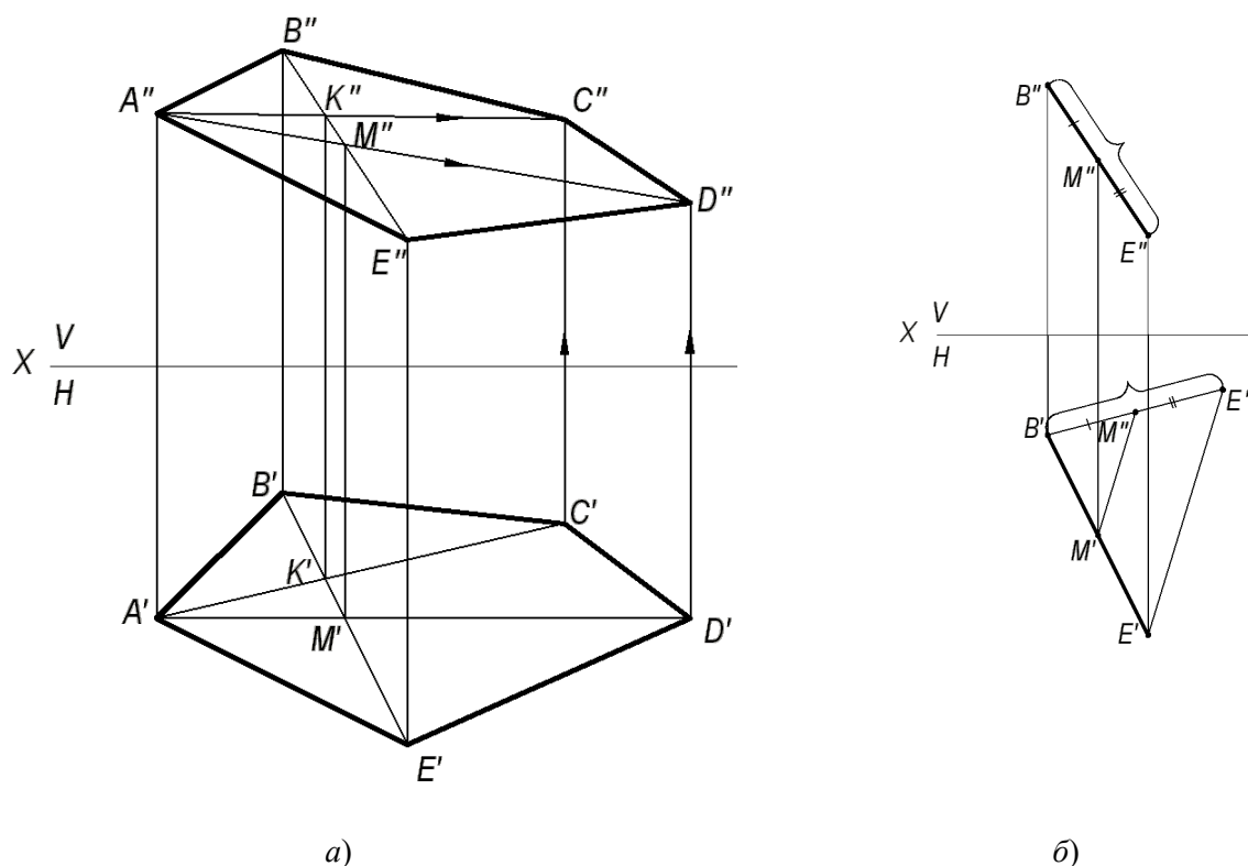
Рис. 1. Построение исходного чертежа многоугольника:
