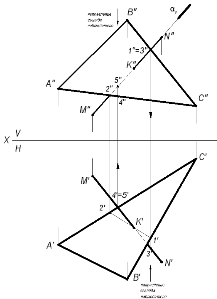
Рис. 2. Построение точки пересечения прямой с плоскостью
