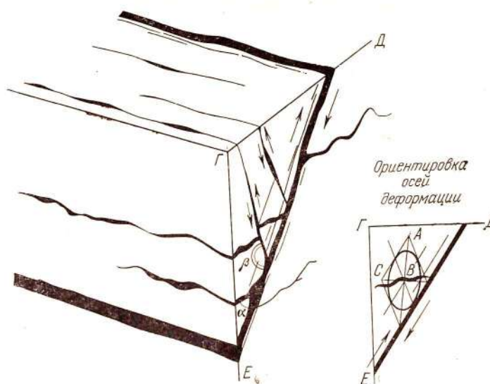
Рис. 12. Схема формирования боковых трещин, оперяющих взброс
