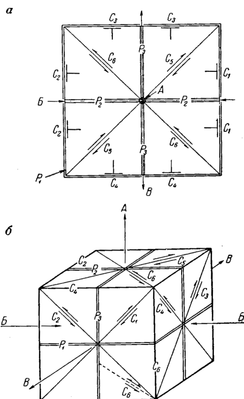
Рис. 3. Основные плоскости деформаций: a – в плане; b – в пространстве. Плоскости: C_1 и C_2 – взброса; C_3 и C_4 – сброса и взброса; C_5 и C_6 – сдвига; P_1 – горизонтального отрыва; P_2 – отрыва; P_3 – сжатия
