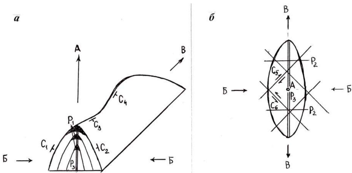
Рис. 4. Положение куба деформаций в складчатых структурах: a – в разрезе, b – в плане
