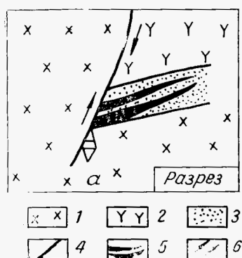
Рис. 52. Схема формирования рудных полей в моноклиальных структурах, в относительно хрупких (а) и относительно пластичных (б) толщах: 1 – порфировые дациты; 2 – порфировые андезиты; 3 – туфоконгломераты; 4 – разломы; 5 – рудные тела; 6 – направление относительных перемещений
