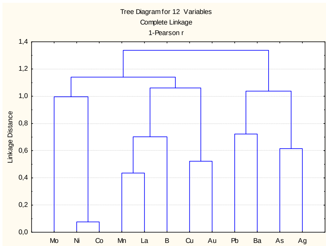
Рис. 5. Дендрограмма
