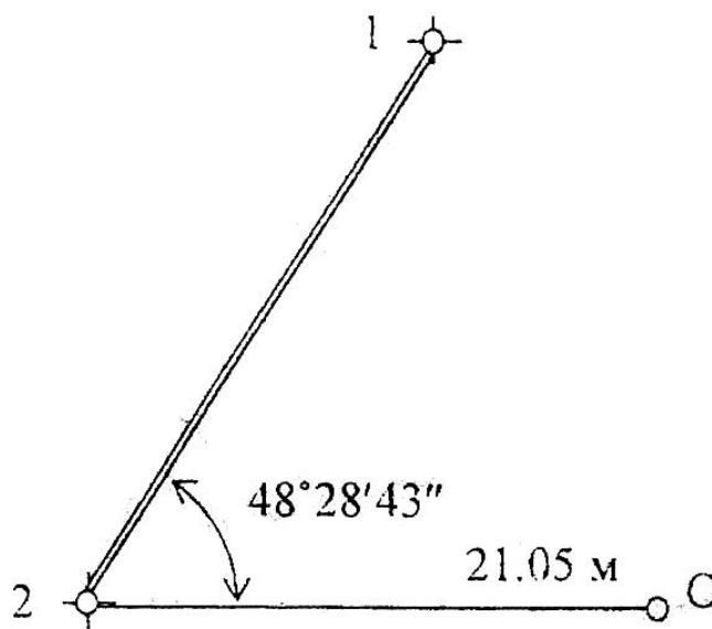
Рис. 7.3 Разбивочный чертеж
