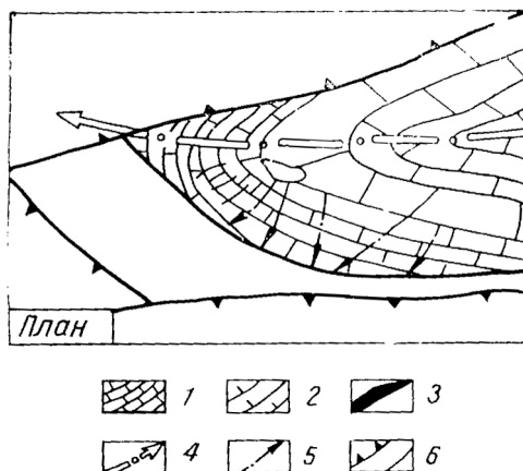
Рис. 1. 54. Принципиальная схема геологического строения рудного поля в периклинальных замыканиях антиклиналей [Атлас]: 1 – слоистые известняки; 2 – массивные известняки; 3 – рудные тела; 4, 5 – оси складок; 6 – разломы
