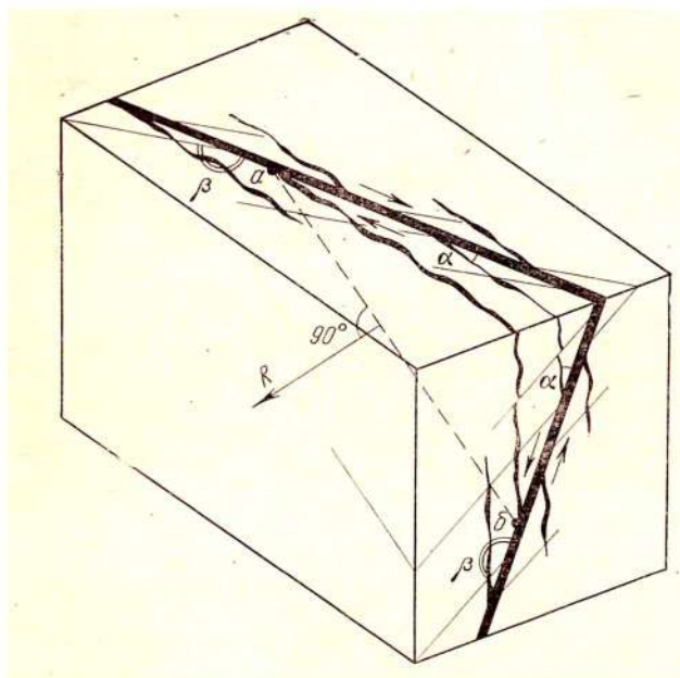
Рис. 12. Схема формирования боковых трещин, оперяющих взброс
