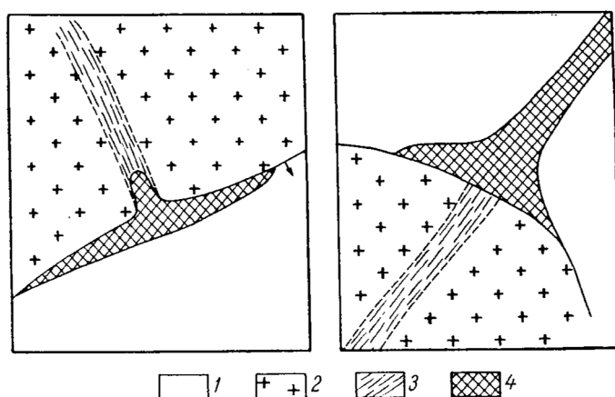
Рис. 50. Шеелитовое оруденение в пересечениях контактов гранитоидных массивов рудоносными разломами. Участок Угат (слева) и месторождение Кумбель (справа): 1 – песчаники и сланцы с прослоями известняков; 2 – граниты; 3 – рудоносные разломы; 4 – шеелитоносные скарны
