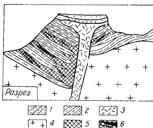
Рис. 1.56. Принципиальная схема рудных полей в синклиналях, осложненных разломами [Атлас]:
