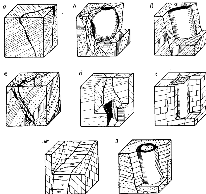
Рис.40. Секущие рудные тела:
