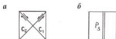
Рис. 1.5. Ориентировка сопряженных трещин в идеально хрупких (а) и в идеально пластичных (б) породах
