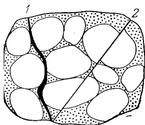
Рис. 1.6. Трещины отрыва (1) и скалывания (2) в конгломератах
