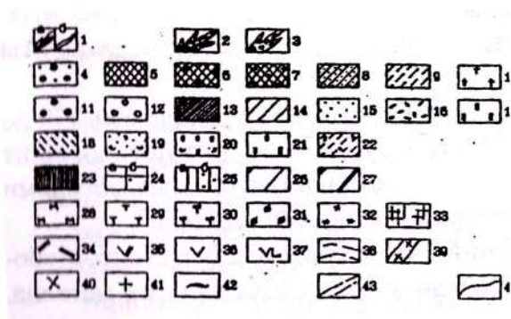
Рис. 1.33. Модель зональности золото-серебряного месторождения Карамкен (Магаданская обл.) [Бен]: 1 – жилы и прожилки: рудные (а), безрудные (б); 2-3 – предрудные изменения: 2 – зоны адуляр-кварц-сульфидного прожилкования, 3 – гидротермальные брекчии; 4-10 – околотрещинные метасоматиты: 4 – существенно кварцевые, 5 – адуляр-кварцевые, 6 – гидрослюдисто-адуляр-кварцевые, 7 – кварц-гидрослюдистые с адуляром, 8 – адуляр-кварц-гидрослюдистые со смектитом, 9 – существенно серицитовые или кварц-серицитовые с карбонатом, хлоритом, 10 – турмалин-кварц-мусковитовые; 11-22 – фации аргиллизитов – вторичных кварцитов: 11 – существенно кварцевая с сульфидами, 12 – монокварцевая, 13 – существенно каолинистая, 14 – кварц-каолинит-диккитовая, 15 – существенно гидрослюдистая, 16 – алунит-кварцевая, 17 – диаспор-кварцевая, 18 – кварц-каолинит-пирофиллитовая; 19 – кварц-гидрослюдисто-смектитовая, 20 – кварц-смектит-хлоритовая, 21 – кварц-хлоритовая, 22 – гидрослюдисто-серицитовая со смектитами, кварцем, карбонатом, хлоритом; 23-27 – фации пропилитов: 23 – цеолит-хлоритовая, 24 (а) – карбонат-альбит-хлоритовая, 24 (б) – карбонат-альбит-серицитовая, 25 (а) – эпидот (пренит)-хлоритовая, 25 (б) – серицит-хлоритовая, 26 – эпидот-актинолит-альбитовая, 27 – роговообманково-биотит-эпидот-альбитовая; 28-33 – прочие изменения: 28 – муско – скарны, 32 – роговики, 33 – калишпатизация; 34-42 – исходные породы: 34 – игнимбриты, 35 – риолиты, риодациты, 36 – дациты, андезидациты, 37 – андезиты, 38 – андезибазальты, базальты, 39 – осадочные породы, 40 – дайки пестрого состава, 41 – габброиды, диориты, 42 – граниты, гранодиориты, 43 – разрывные нарушения, 44 – фациальные границы
