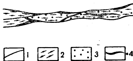
Рис. 1.59. Схема размещения оруденения в сложном разломе (план) [Карамазар]: 1 – линии разрывных нарушений; 2 – зона дробления пород; 3 – вкрапленное оруденение; 4 – рудные тела
