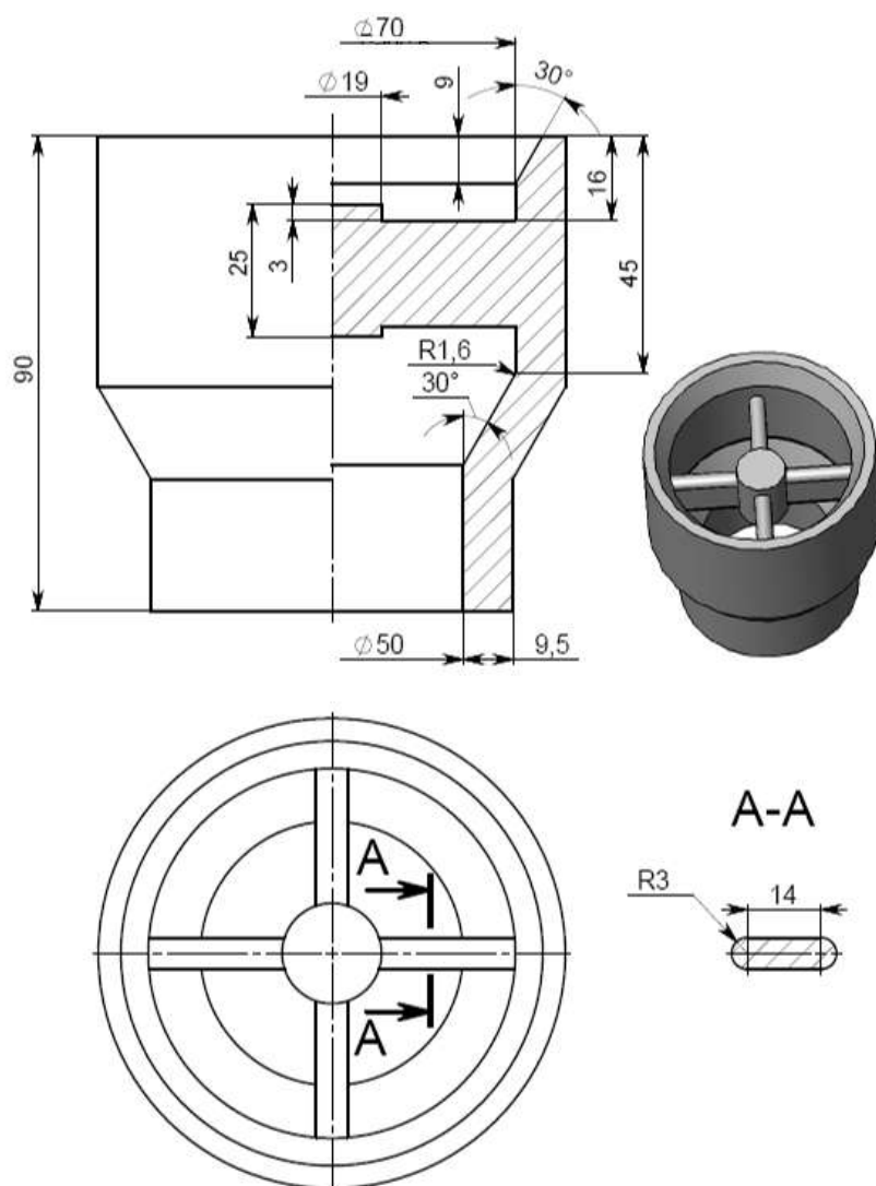
Рис. 2. Направляющая
