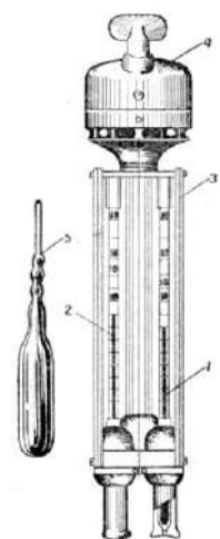
Рис. 3.3 Психрометр Ассмана
