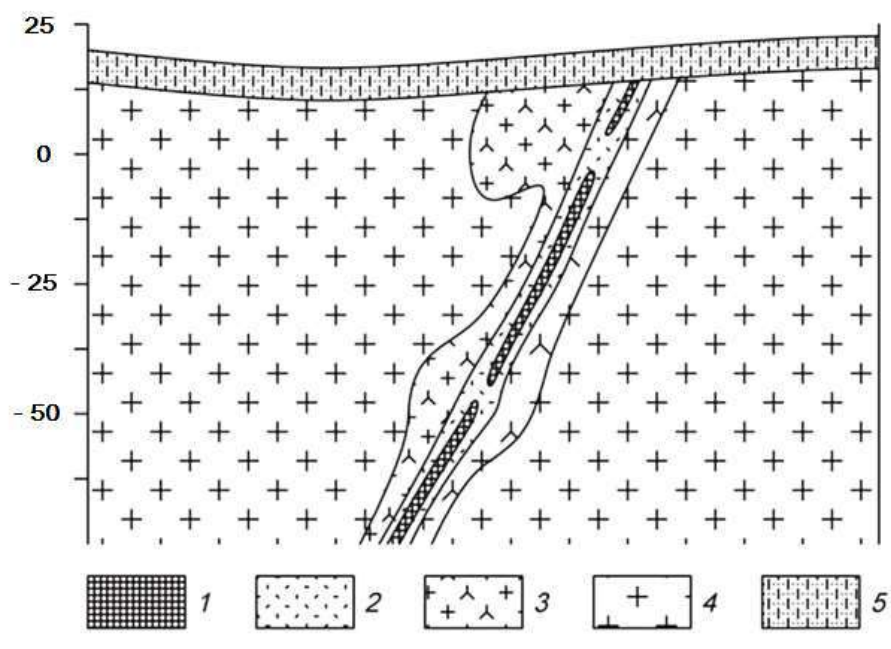
Схематический геологический разрез кварц-сульфидного медного месторождения. 1 – кварц-магнетит-халькопиритовые руды, 2 – прожилково-вкрапленные руды, 3 – гидротермально измененные граниты, 4 – биотитовые граниты, 5 – известковистые песчаники.
