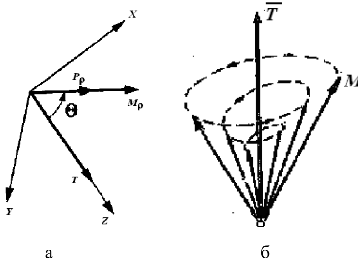
Рис. 33. К выводу уравнения прецессии протона в магнитном поле
