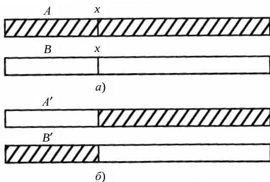
Рис. 3.3. Схема кроссинговера:
